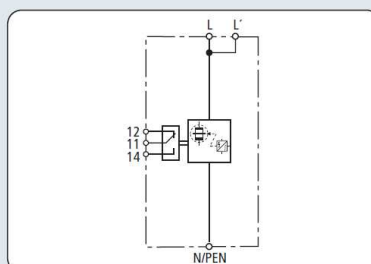
Schéma de principe du circuit DBM 1 440 FM
